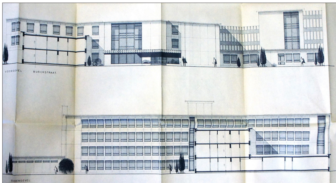
Orthogonale projectie van de voorgevels in het laatste voorontwerp van de uitbreiding ziekenhuis, 13 juli 1973 door J.M. Peeters.
